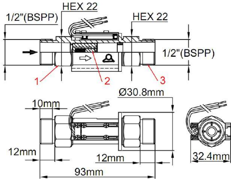
1: 1/2" BSPP进水口 2: 流量探测活塞 3: 1/2" BSPP出水口
